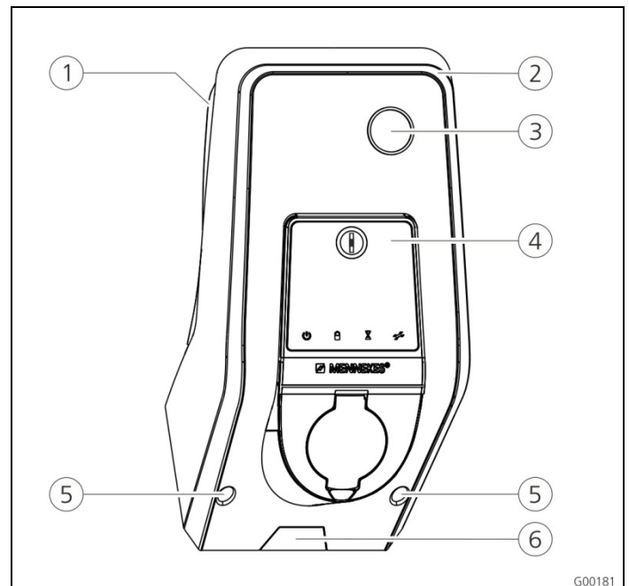
Abb. 4: Frontansicht (Beispiel)
