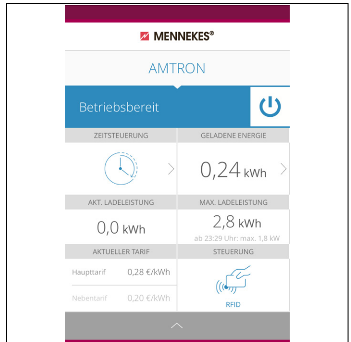
Abb. 7: Charge APP (Beispiel)
