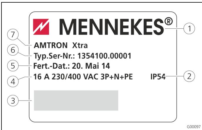
Abb. 2: Typenschild (Beispiel)
