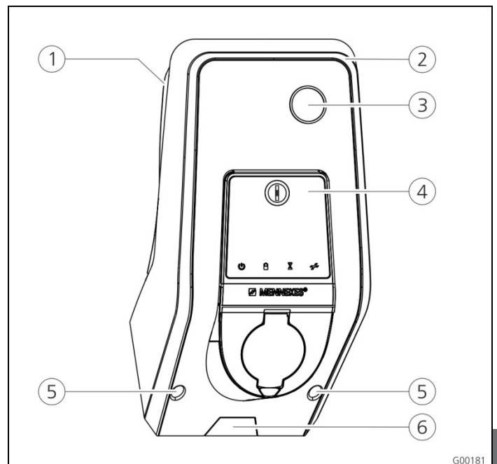
Afb. 4: Frontaanzicht (voorbeeld)
