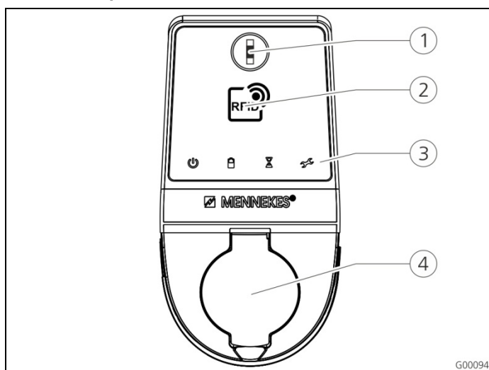
Afb. 6: Frontpaneel (voorbeeld)
