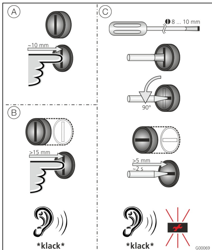
Fig. 8 : touche multifonctions
