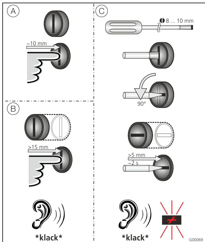
Abb. 8: Multifunktionsstaster
