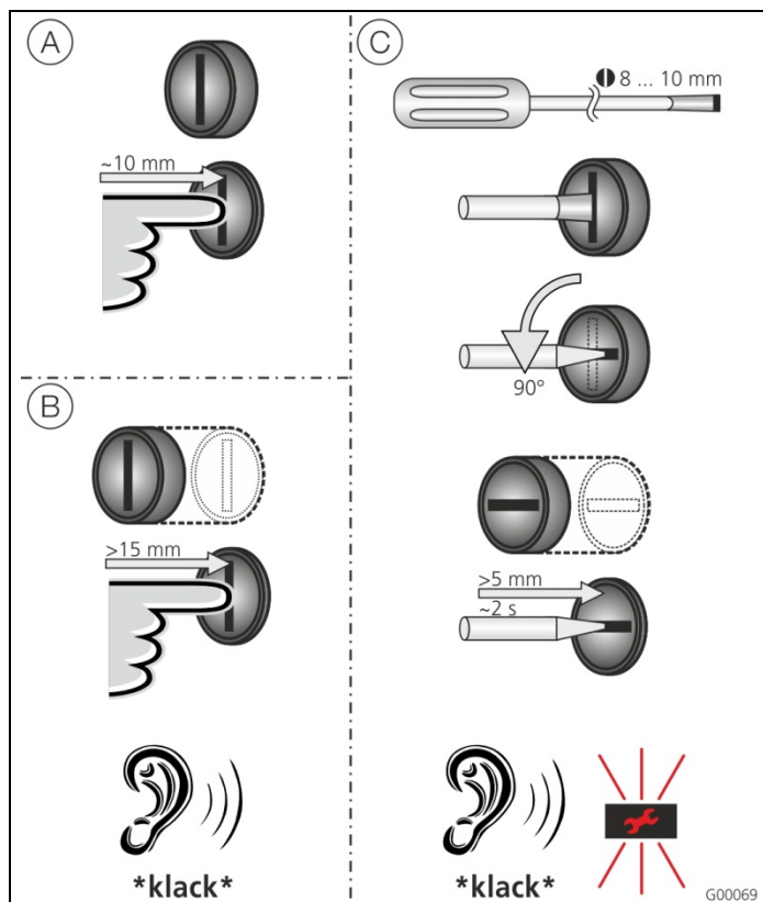
Afb. 8: Multifunctietoets
