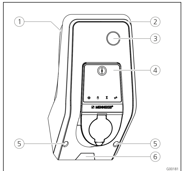
Fig. 4 : vue frontale (exemple)
