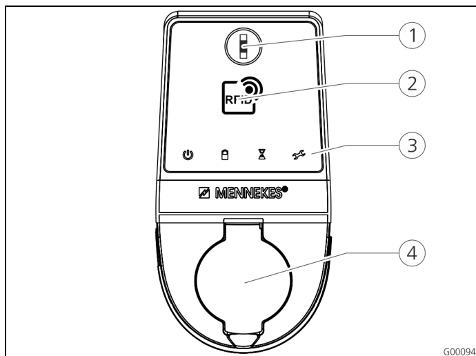
Fig. 6: Frontpanel (eksempel)
