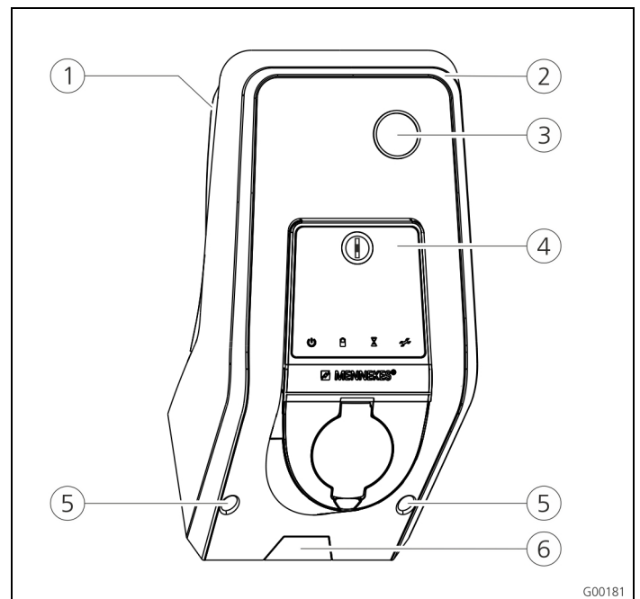
Fig. 4: vista frontale (esempio)
