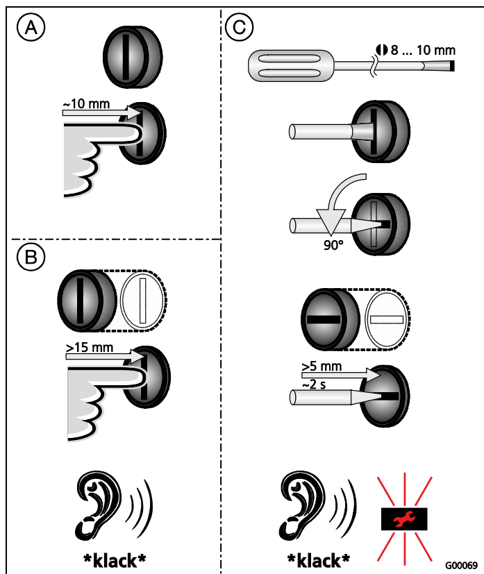
Fig. 8: tasto multifunzione
