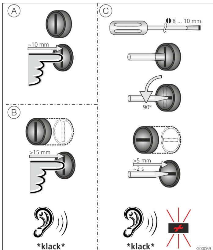
Fig. 8: Multifunksjonsknapp
