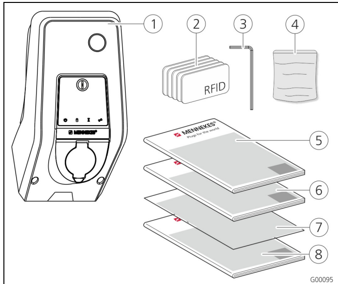
Abb. 3: Lieferumfang
