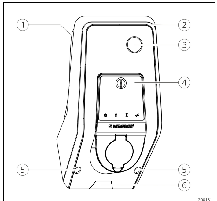
Fig. 4: Sett forfra (eksempel)
