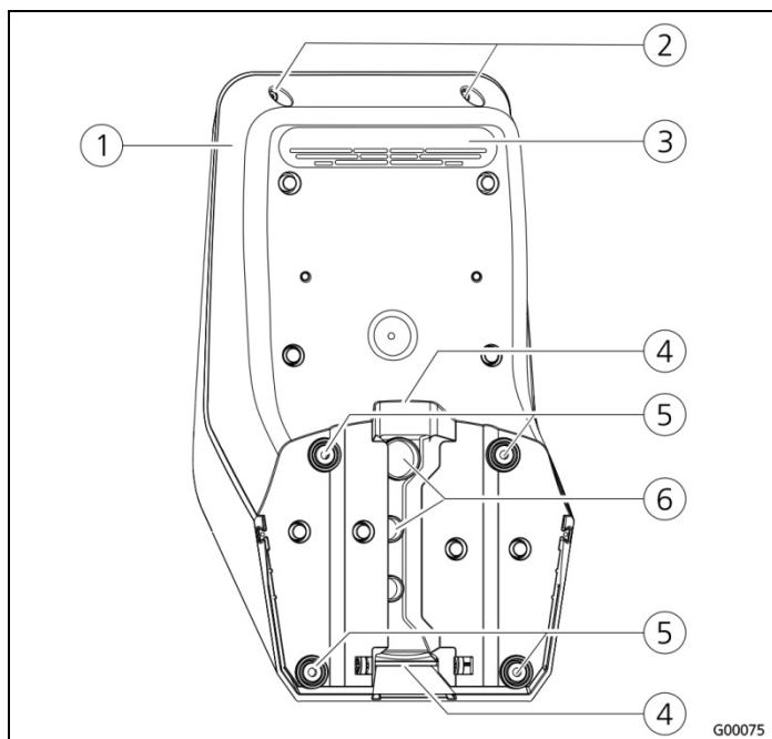
Afb. 5: Achteraanzicht (voorbeeld)
