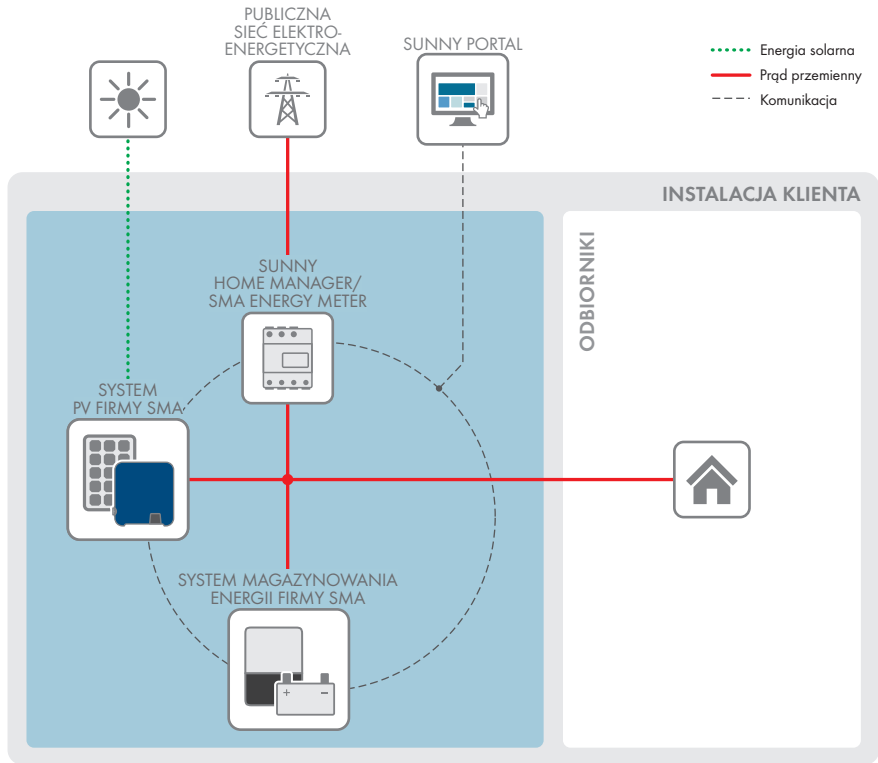
Ilustracja 3: Budowa systemu
