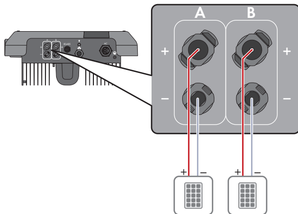
Ilustracja 10: Widok przyłącza przy normalnej eksploatacji
