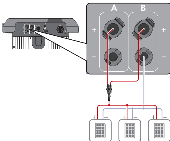
Ilustracja 11: Widok przyłącza przy równoległym podłączeniu wejść DC A i B
