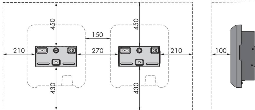
Ilustracja 8: Zalecane odstępy (wymiary w mm)
